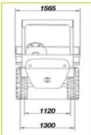
DH-160 P
